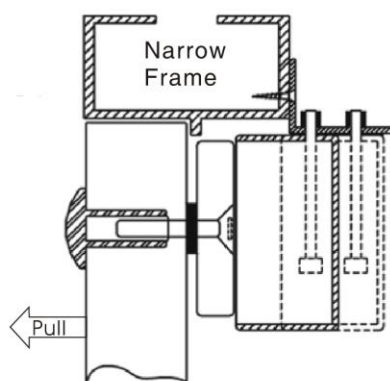
Narrow door frame(swing out)
